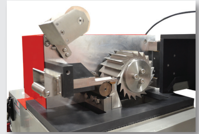
Upper Feedroll Pivots for quick access Cubierta de Bisagra Fácil de Abrir
