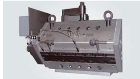
SG 450C die head
